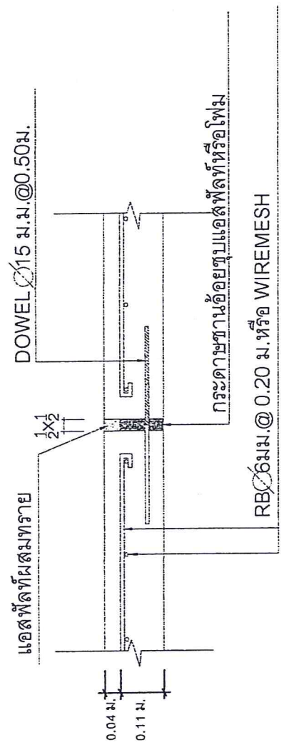
ขยายรอยต่อขาดจากกัน EXPANSION JOINT
