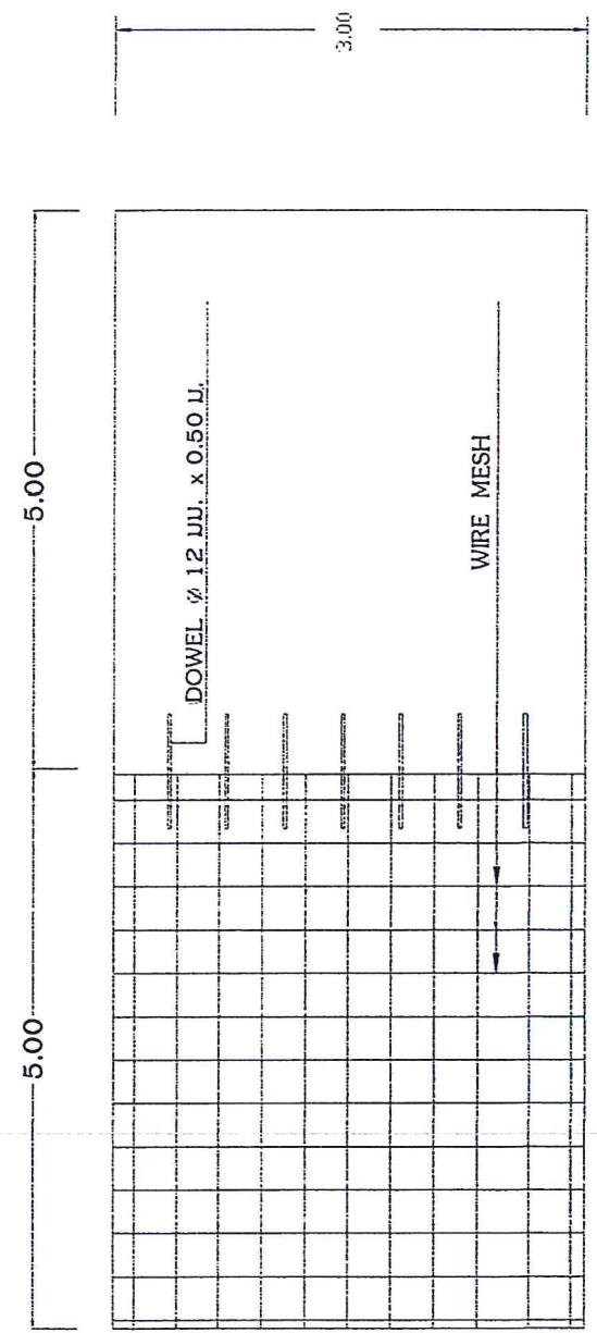
แปลนแสดงการผูกเหล็ก
